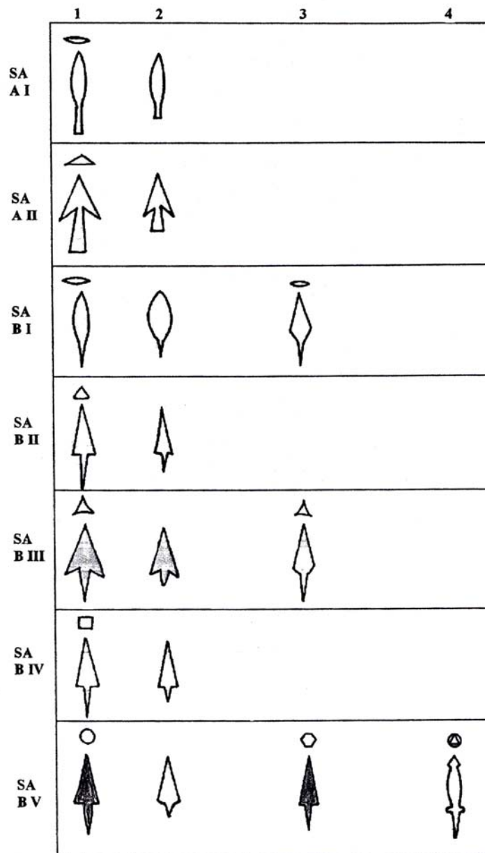
Fig. 8. Schemă cu înscrierea vârfurilor de săgeată din fier de la Potaissa/Turda în tipologia generală.
